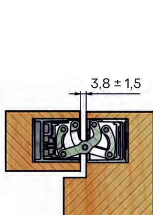
0° (zavřené dveře)
