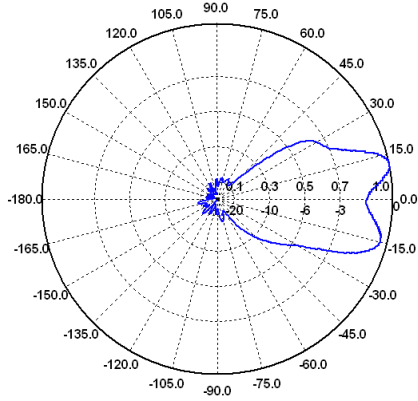
E-Ebene / E-Plane 1.4 GHz
