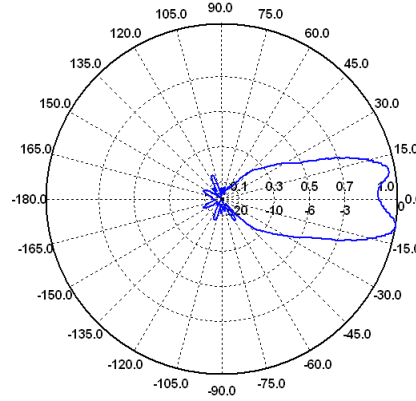
H-Ebene / H-Plane 1.4 GHz
