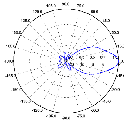
H-Ebene / H-Plane 800 MHz
