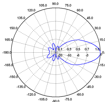
H-Ebene / H-Plane 700 MHz
