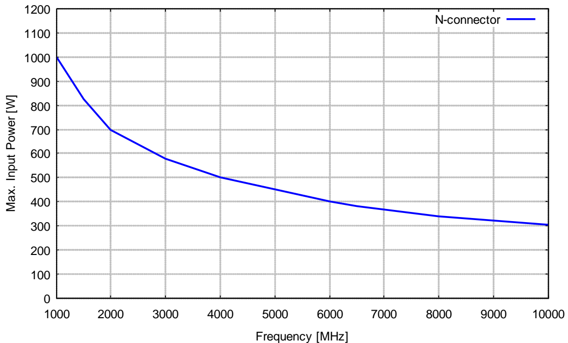
Maximale Eingangsleistung
