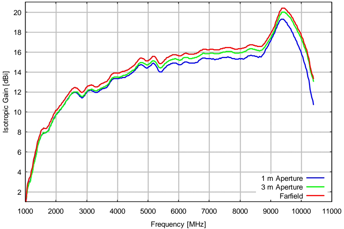
Isotropgewinn
