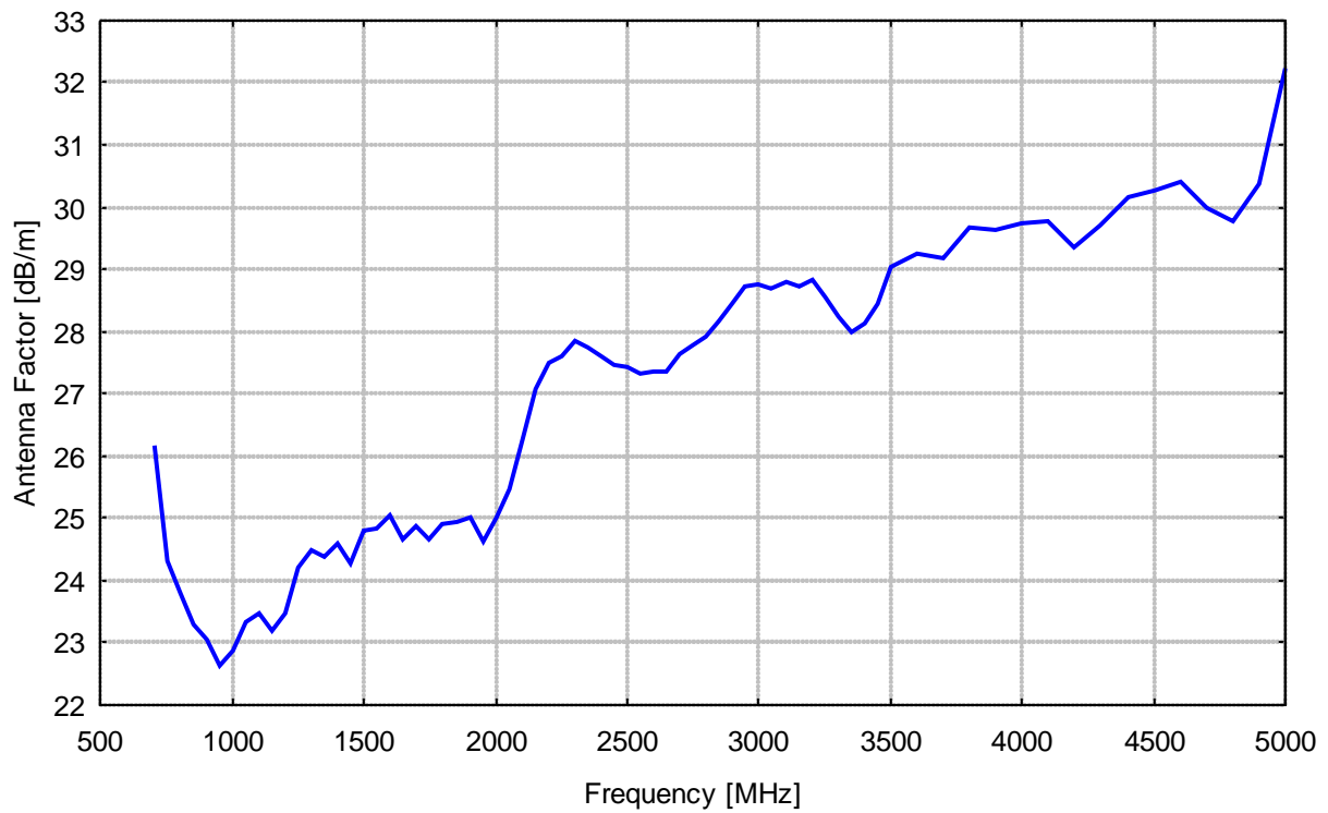
Antennen-Wandlungsmaß
