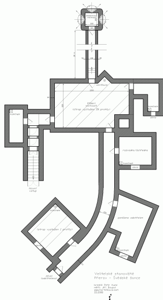
Půdorys objektu pozorovatelny civilní obrany vybudované v první polovině 50. let 20. století v místech původní reduty švédského tábora z roku 1643. Kresba P. Kunc, zaměření J. Doupal.
