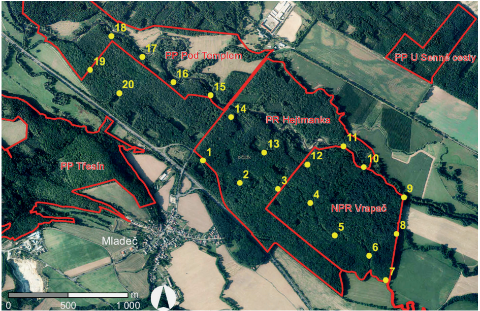
Obr. 1 / Fig. 1: Zobrazení monitorovaných bodů na transektu Vrapač (A) a Litovelské luhy (B) (červeně jsou vyznačeny hranice maloplošných zvláště chráněných území). / Localisation of counted points at Vrapač (A) and Litovelské luhy (B). Red line – boundaries of nature reserves.
