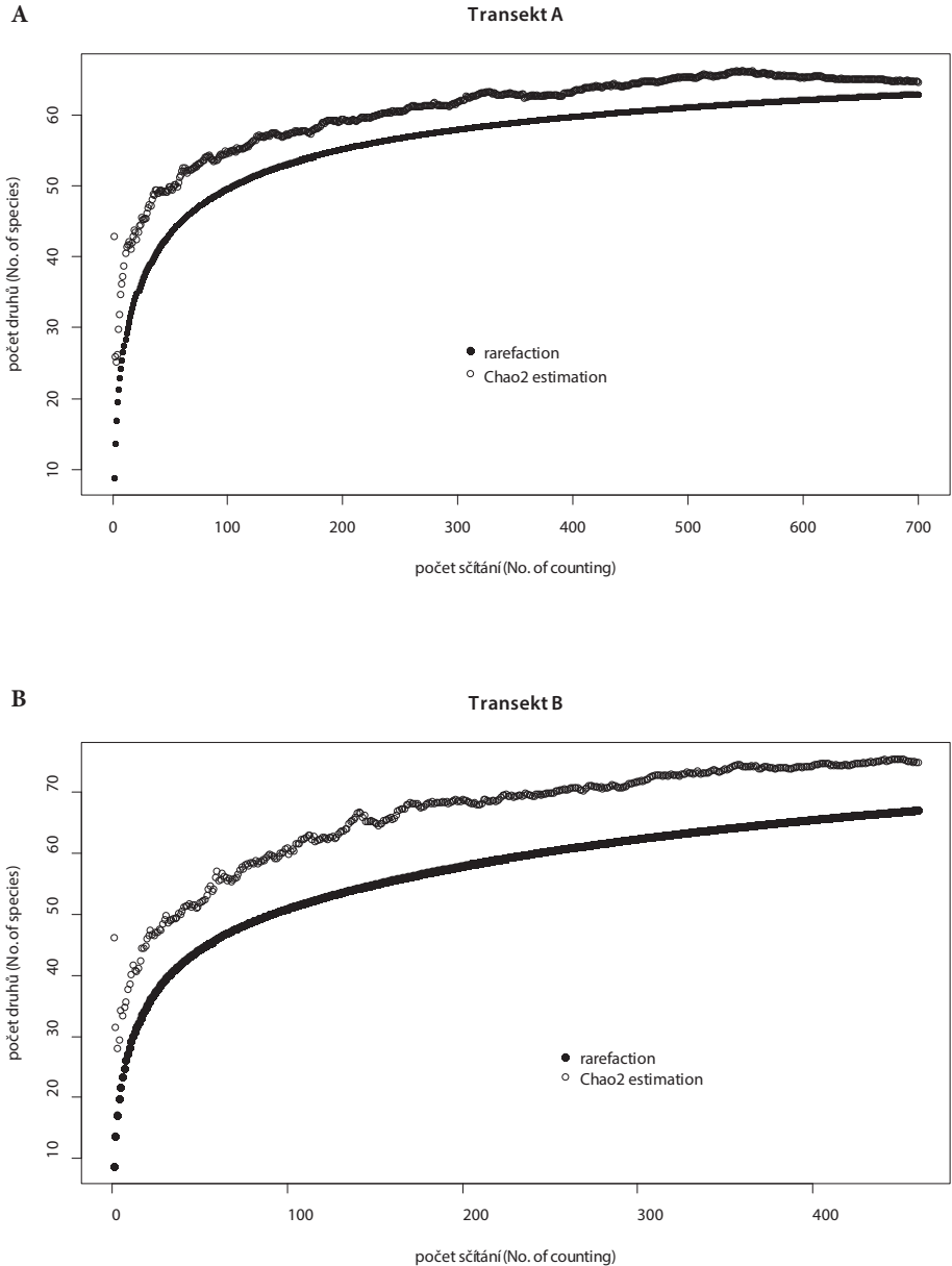
Ob. 2 / Fig. 2: Vztah sčítacího úsilí a počtu zaznamenaných druhů na transektu Vrapač (A) a Litovelské luhy (B). Křivky celkové druhové bohatosti (odhadnuté metodou rarefakce) jsou znázorněny plnými body, křivky odhadované druhové bohatosti (Chao2 extrapolace) prázdními body. / Relation between counting effort and the number of detected species at Vrapač transect (A) and Litovelské luhy (B). The curve of total species richness (estimated by rarefaction method) show solid circles, curves of estimated species richness (Chao2 extrapolation) by empty circles.
