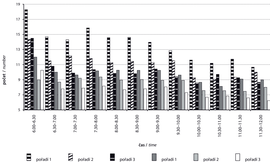
Obr. 3 / Fig. 3: Průměrný počet zjištěných jedinců (šrafované sloupce) a druhů (plné sloupce) v jednotlivých časových intervalech s rozlišeným pořadím sčítání v roce (polovina dubna, května, června) – souhrn výsledků z obou bodových transektů Vrapač a Litovelské luhy./ The average number specimens (shaded columns) and species (solid columns) in different time intervals with different counts of the year (mid April, May and June).
