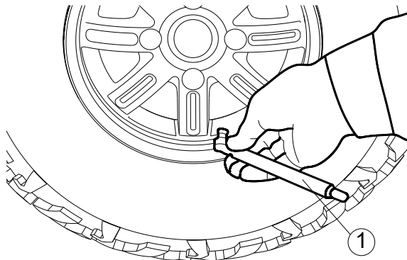
1. Manometr
