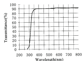
Spektrální charakteristika skel, d=0.15 mm
