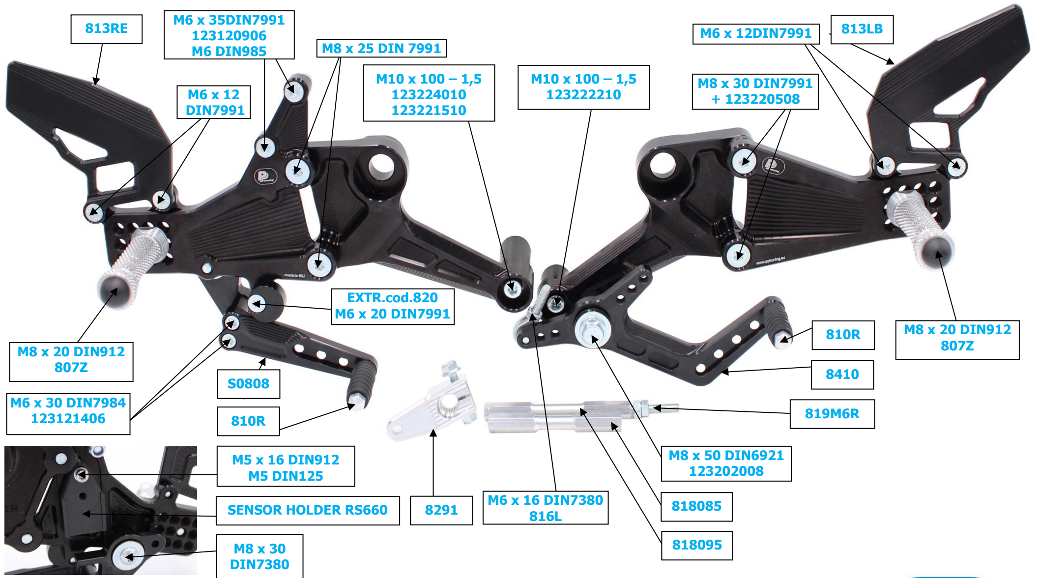
APRILIA RS660 2021 – Part nr. 506
